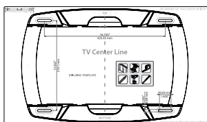
Template (Qty 1)
